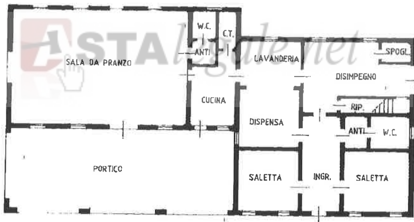
PIANTA PIANO TERRA h. 2.80
