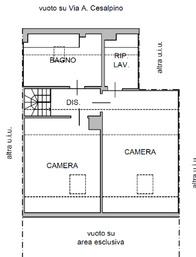
PIANTA PIANO PRIMO-SOTTOTETTO (2° f.t.)
